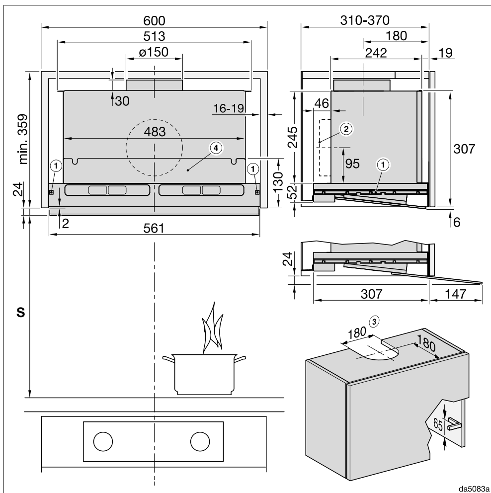
Slika 1: DAS 4640 u ormariću širine 600 mm.
